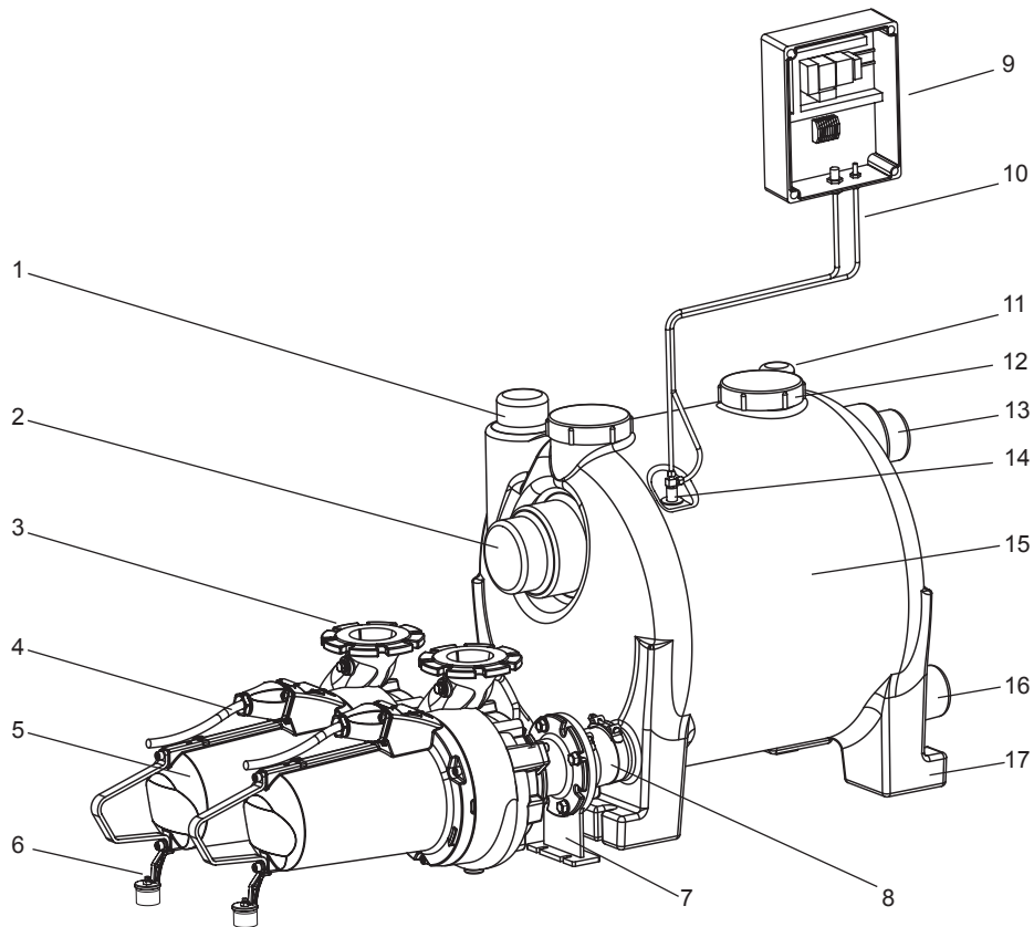
Abb. 2: Aufbau der Hebeanlage
