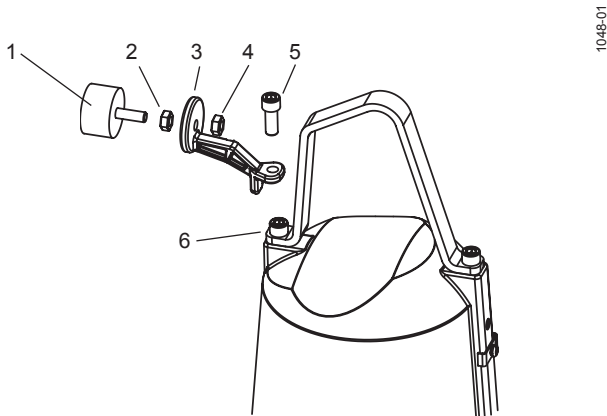
Abb 6: Montage der Kopfstütze
