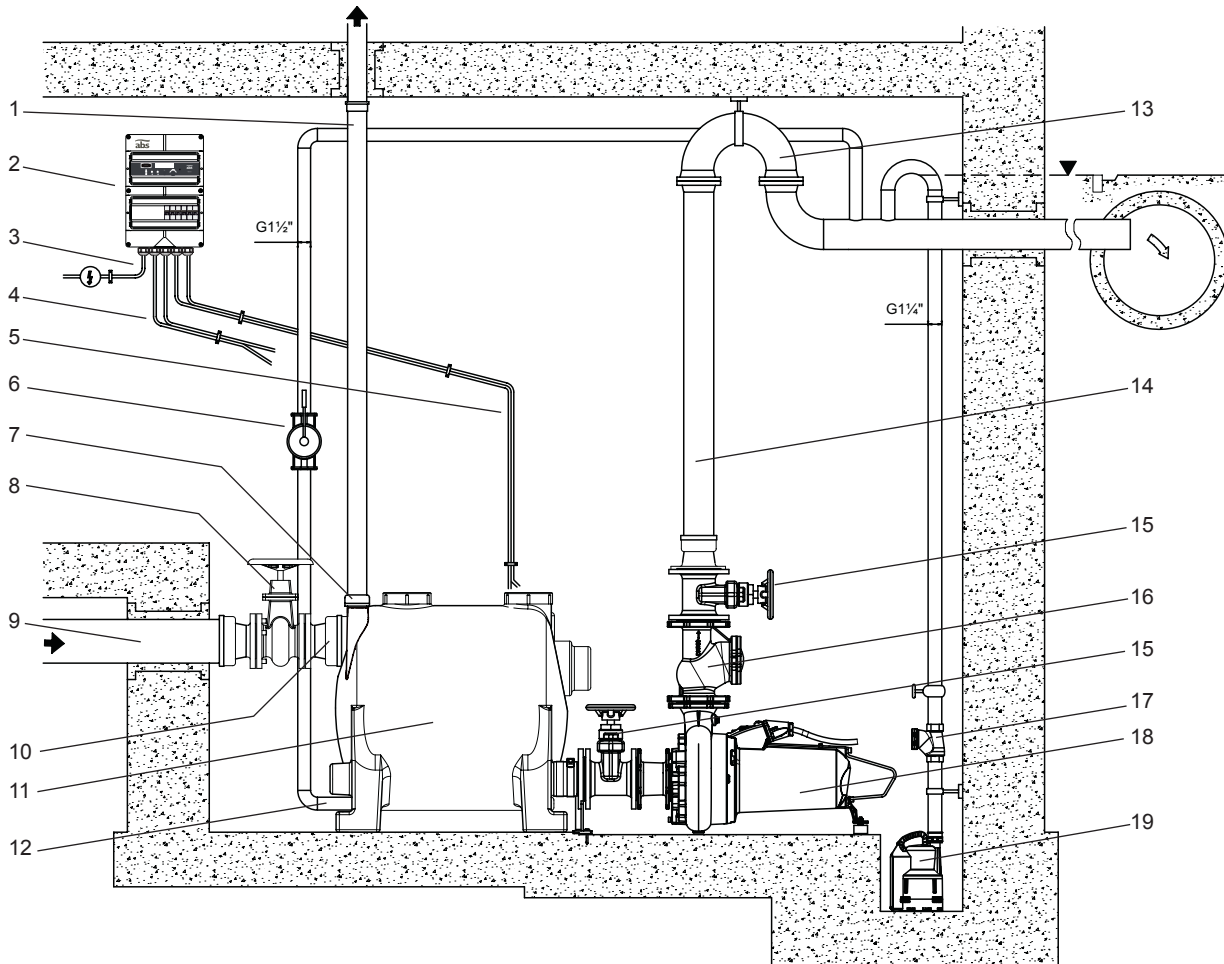
Abb. 3: Installationsbeispiel
