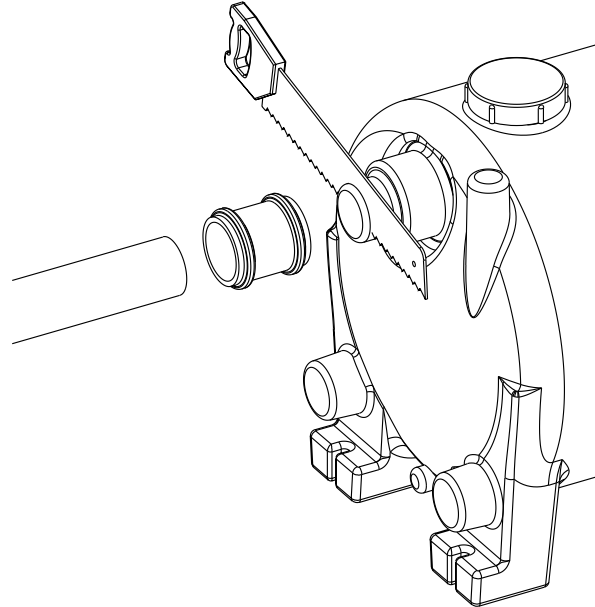
Abb. 5: Öffnen der Anschlüsse am Sammelbehälter
