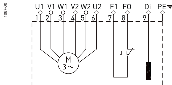
Abb. 11: Schaltpläne XFP 80C, 100C & 100E
