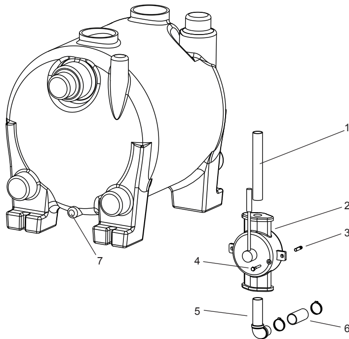
Abb. 12: Installation der Handmembranpumpe
