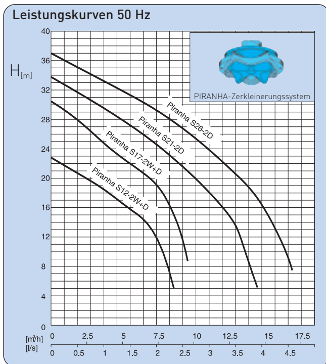
H = Gesamtförderhöhe Q = Förderstrom Kennlinien nach ISO 2548/C
